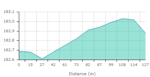
Coupe DD' (pente moyenne de 2%)
