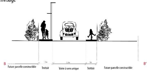
Profil envisagé
