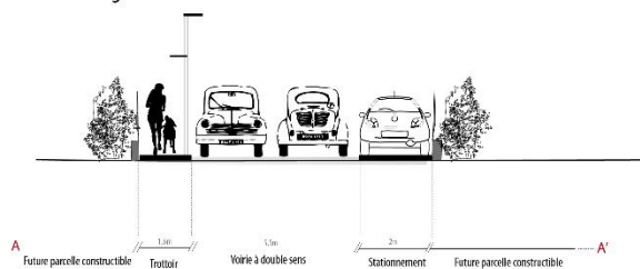
Profil envisagé
