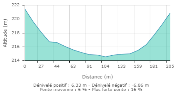
Coupe CC'
